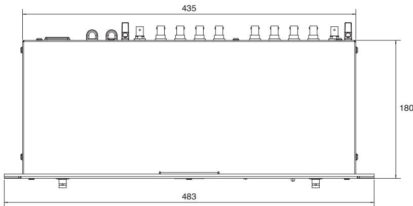
上面図
