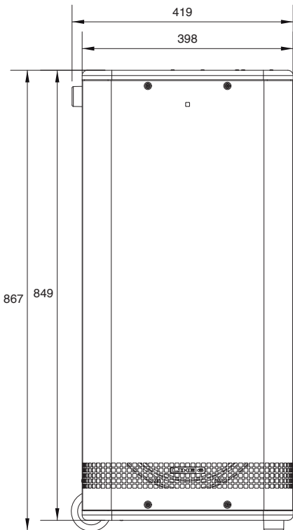
正面図
